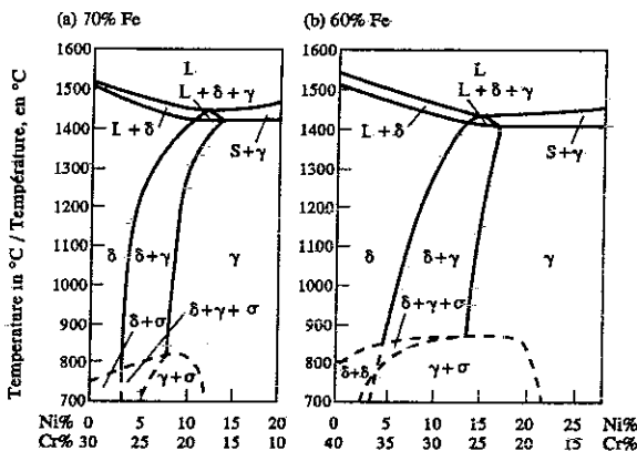
Fig. 1. Pseudo-binary constitution diagrams Fe-Cr-Ni [2]/ Diagrammes de constitution pseudo-binaires Fe-Cr-Ni [2]
