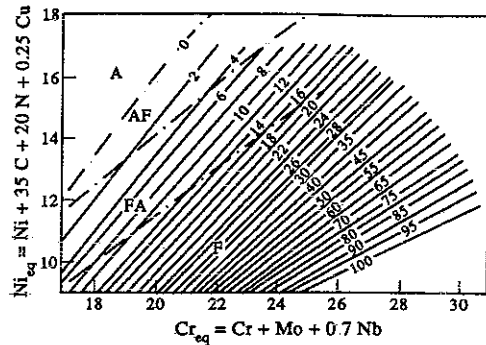
Fig. 2. WRC 1992 Diagram [7]/Diagramme de constitution WRC 1988 [7]
