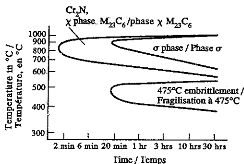
Fig 4. ITT diagram for parent material type 22% Cr duplex stainless steel (UNS 31803)/Diagrammes TTT du métal de base en acier duplex à 22% Cr (UNS 31803)
